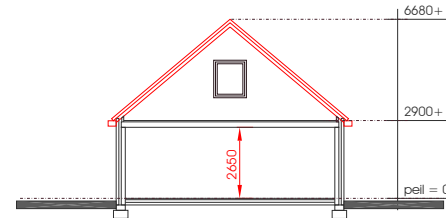
doorsnede
