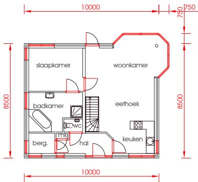
begane grond
