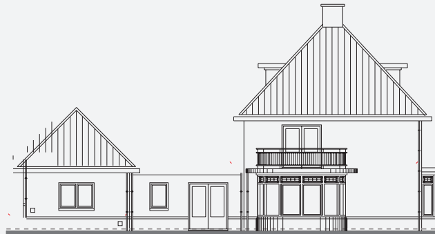
linkerzijgevel
