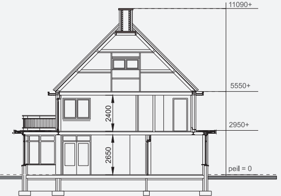
doorsnede
